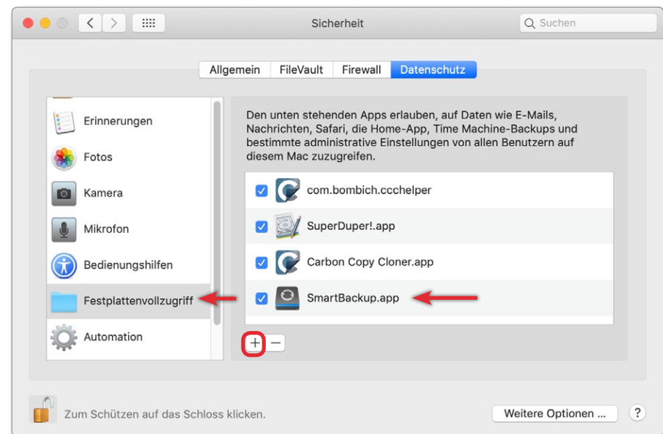
Abb. 9: Man sollte unter macOS 10.14 SmartBackup den Festplattenvollzugriff gewähren.
